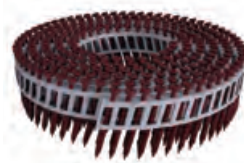
Žblji z navojem v kolutu 16° (črni, rdeči) Pakiranje: 2000 kosov
